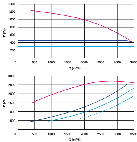
Caudal y potencia VEX550-C4
