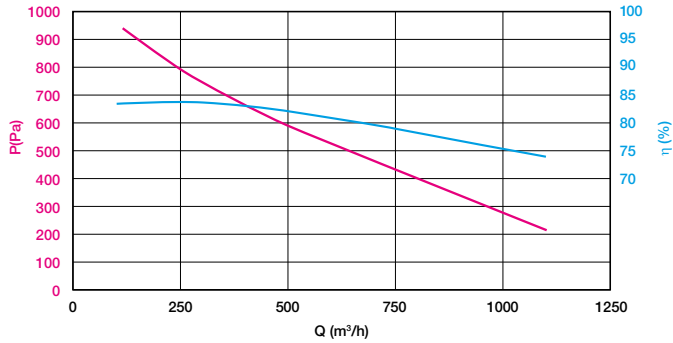
Características aerúlicas VEX720T
