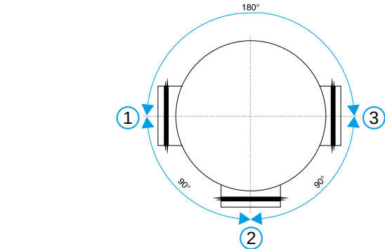
Esquema dimensiones Colector Conexión de Planta con juntas
