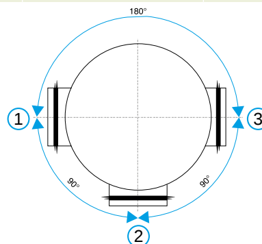
Esquema dimensiones Colector Conexión de Planta con juntas
