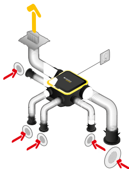
Instalación Easyhome Auto Compact con bocas BIP y conductos Algaïne
