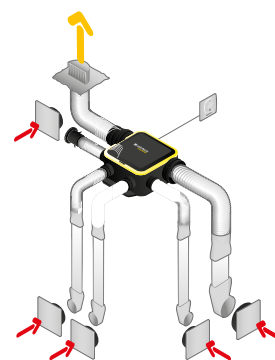
Instalación Easyhome Auto Compact con bocas ColorLINE® y Miniconducto
