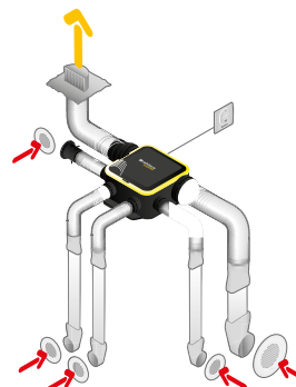
Instalación Easyhome Auto Compact con bocas BIP® y Miniconducto
