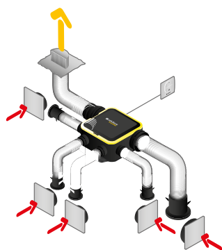
Instalación Easyhome Auto Compact con bocas ColorLINE® y conductos Algaïne
