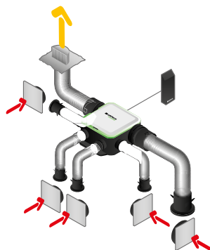
Instalación con conductos flexibles Algaire
