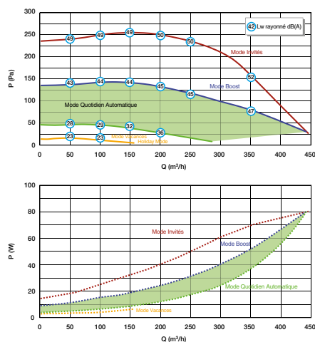
Curva aeráulica y acústica EasyHOME PureAIR COMPACT Connect
