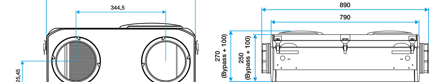
Echangeur vue piquages
