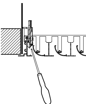
Difusor de impulsión con fijación S3
