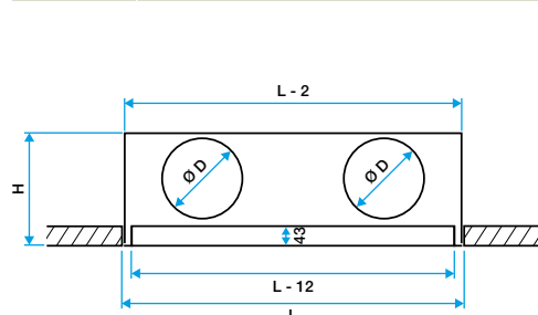
Lined S Slim avec plénum. Fixation S2 ou S3
